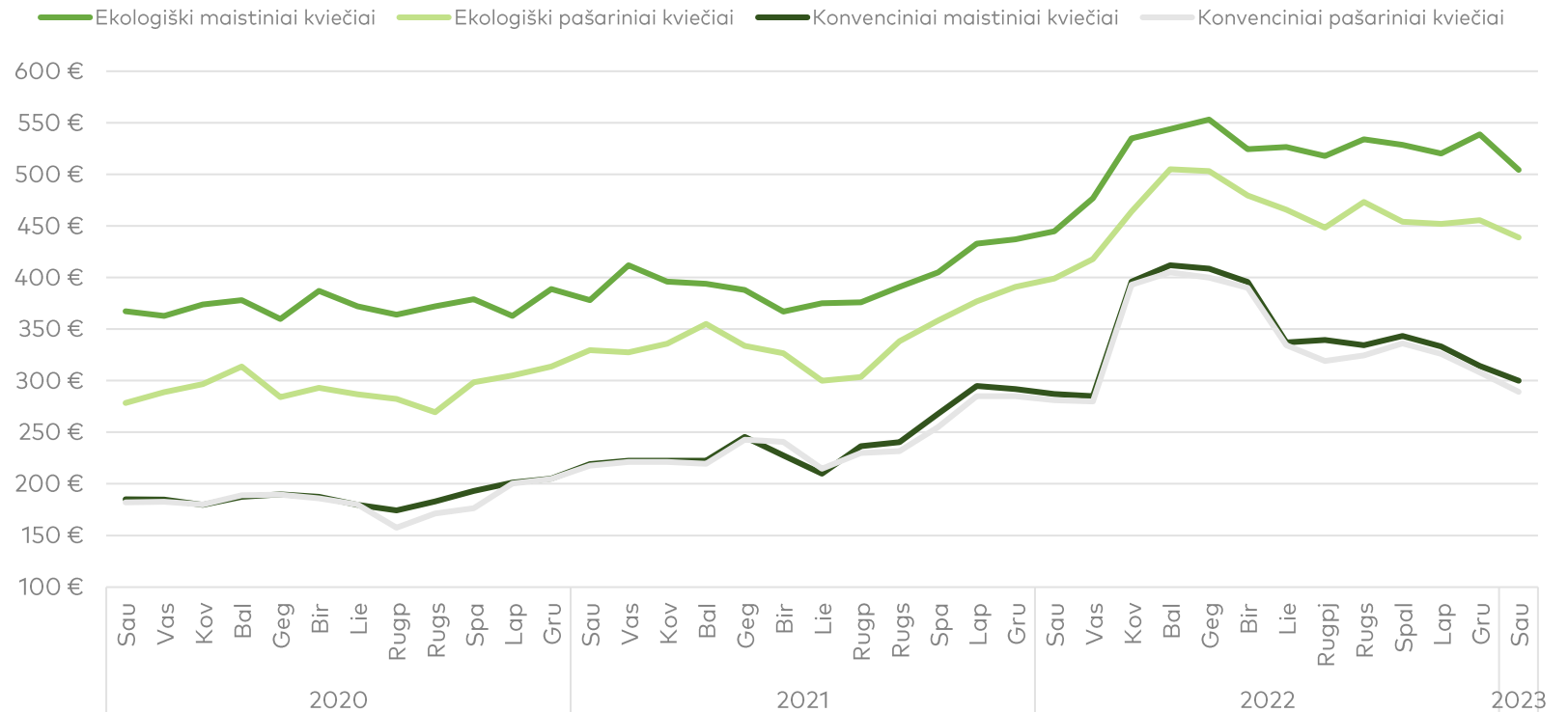
Ekologinių ir konvencinių kviečių kaina Vokietijoje*, Eur/t
